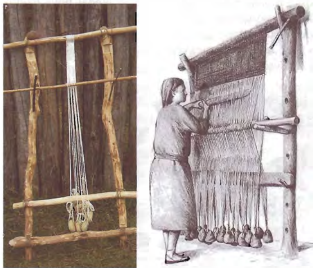
▲ Obr. 16 Replika vertikálního tkalcovského stavu a kresebná rekonstrukce práce na něm
