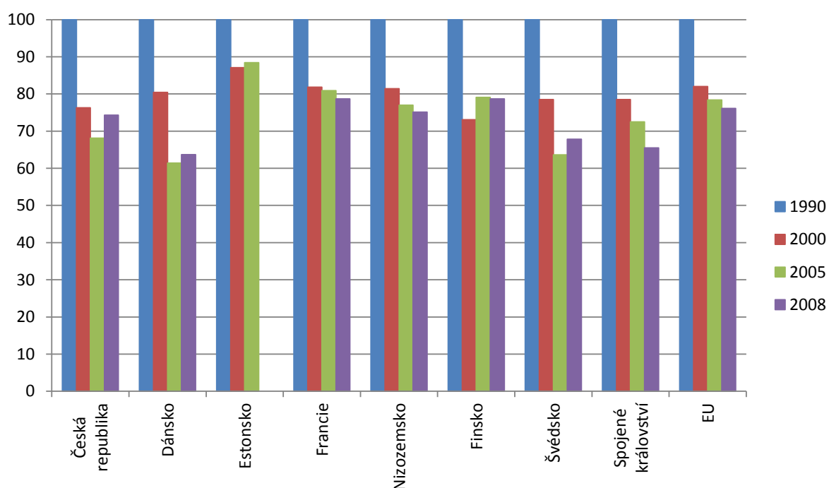
Graf IV.C.2 Indikátor ptáků zemědělské krajiny, mezinárodní srovnání, 1990, 2000, 2005, 2008
