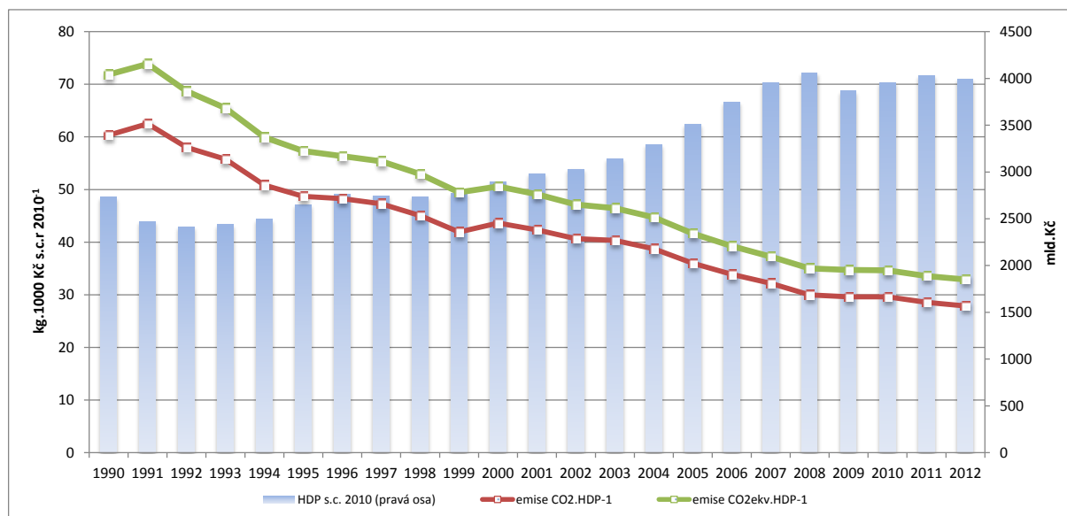
Graf V.G.2: Agregované emise skleníkových plynů a emise CO 2 na jednotku HDP [kg CO 2 ekv. 1000 Kč s.c.r 2010 -1 , mld. Kč], ČR, 1990-2012
