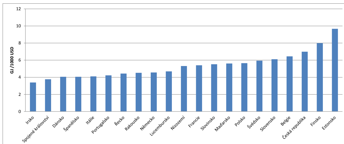
Graf II.E.2: Energetická náročnost HDP, mezinárodní srovnání, 2013
