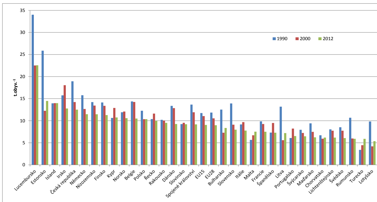
Graf V.G.3: Agregované emise skleníkových plynů na obyvatele[t CO 2 ekv.obyv. -1 ] mezinárodní srovnání, 1990, 2000, 2012
