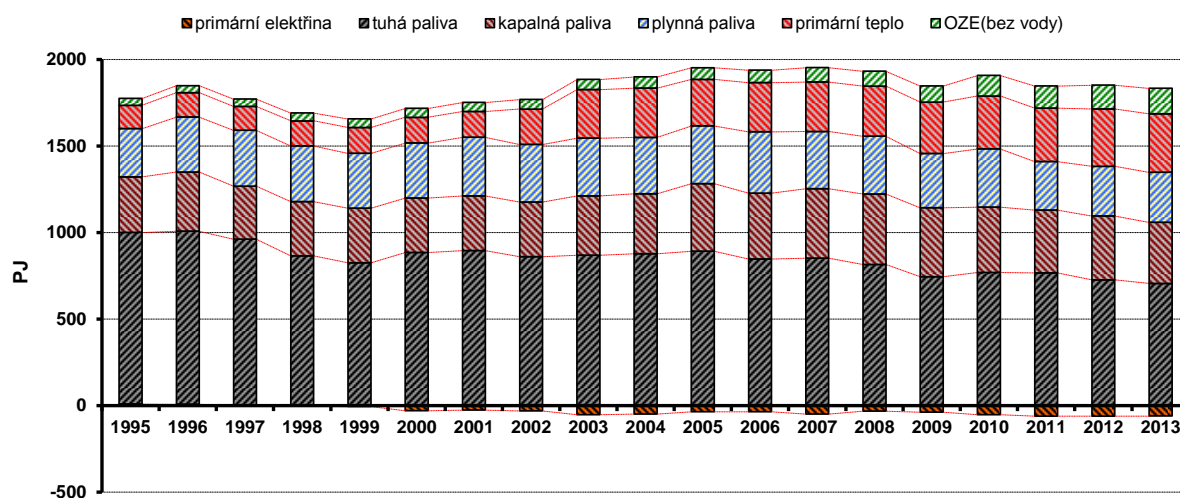
Graf II.F.1: Primární energetické zdroje, Česká republika, 1995-2013 10
