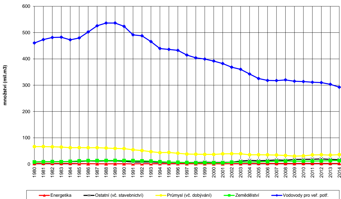
Graf II.I.2: Odběry podzemních vod, ČR, 1980-2014
