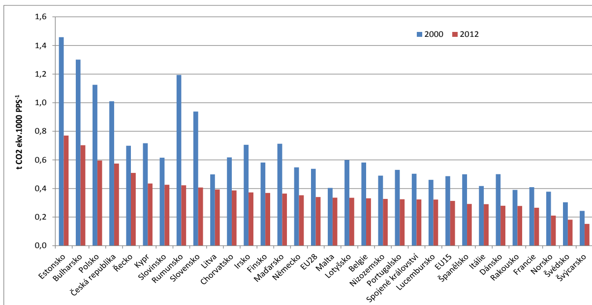
Graf V.G.4: Agregované emise skleníkových plynů na jednotku HDP [t CO 2 ekv.1000 PPS -1 ], mezinárodní srovnání, 2000, 2012
