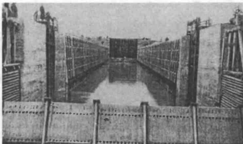
В шлюзе поднят ремонтный затвор
