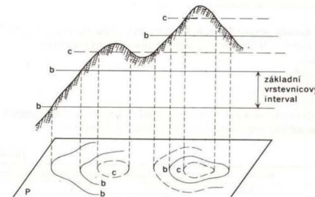
Obr. 2-21 Princip vrstevnic
