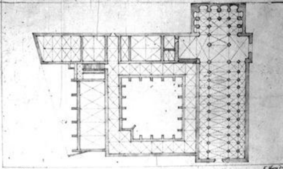
Chrám i klášter Zbraslavský před r. 1420. Podle starých výkresův nálezcých 1850 v matricei cís. fornika Vestala a Hlaváček Měšťanských.
