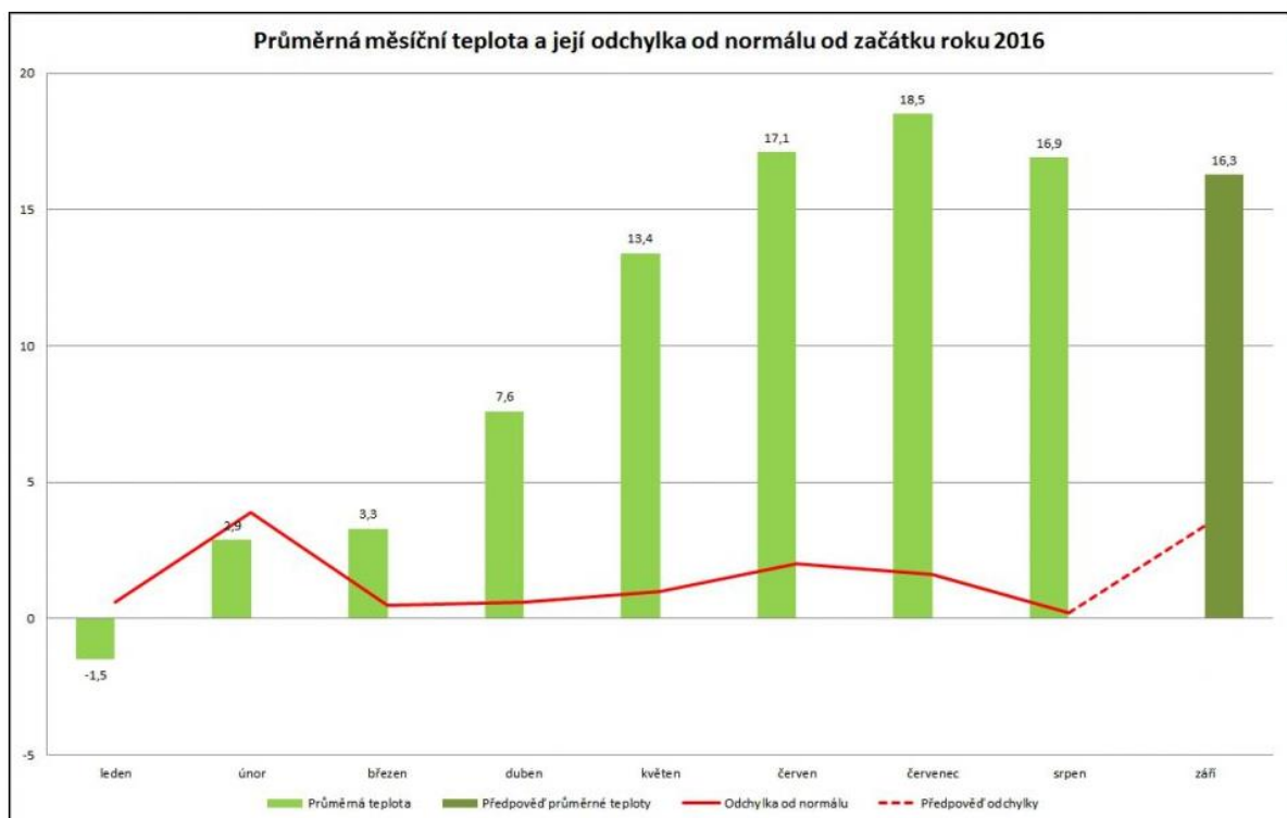
Průměrná měsíční teplota od začátku roku a její odchylka od normálu. Zdroj: ČHMÚ
